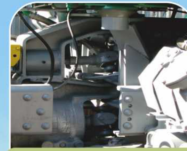
Усиленный вертикальный шарнир соединения полурам ①,②
